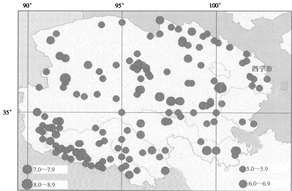
图 1-1-2 青海省地震震中分布图
