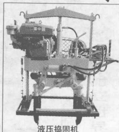
液压捣固机
