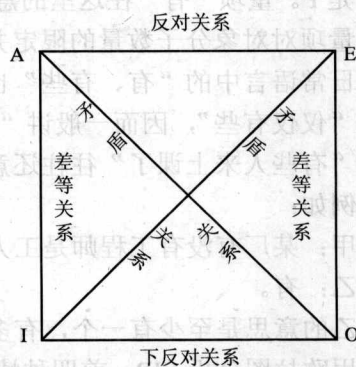
图 1-6 逻辑方阵
