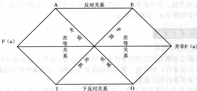
图 1-7 对当方阵
