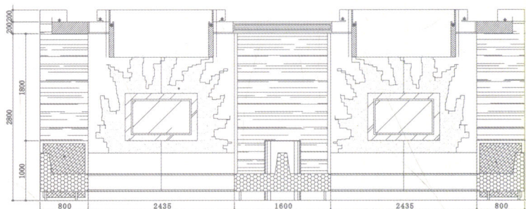
总统套房立面图
