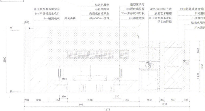
标准客房立面图
