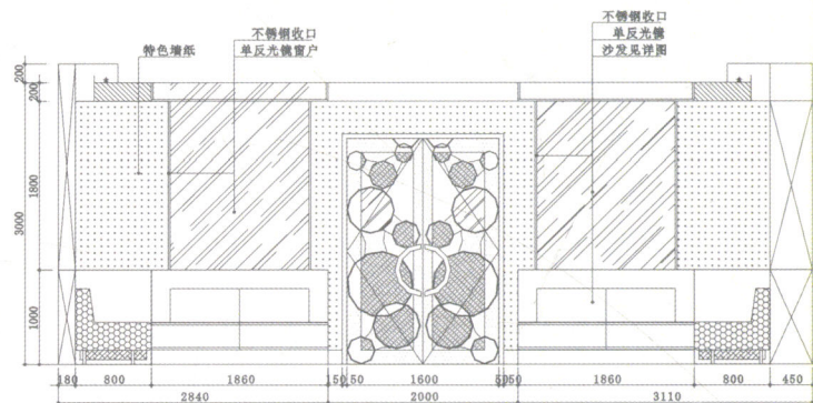
总统套房立面图
