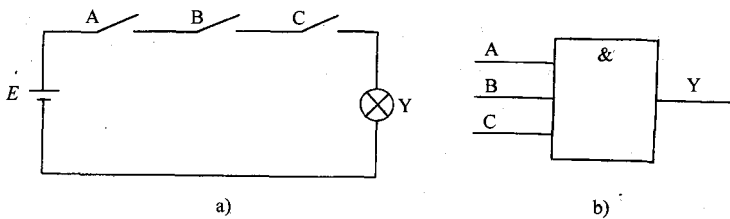
图 10-1 与逻辑的示意电路和逻辑符号 a) 由开关组成的与逻辑电路 b) 与逻辑符号
