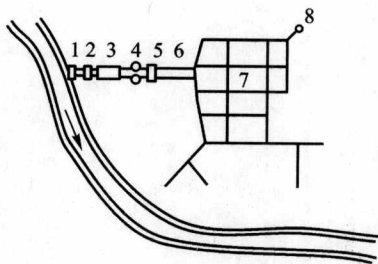
图 2-2 用地表水源的城镇给水系统示意图
