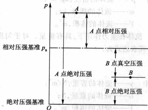
图 1-1 压强关系图
