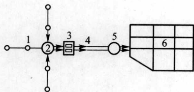
图 2-1 用地下水水源的城镇给水系统示意图
