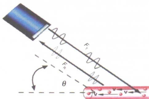
图1-1-1 多普勒效应示意图
