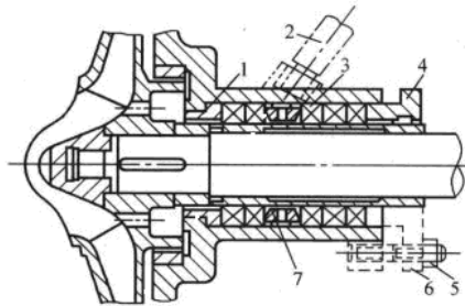
图 2-7 填料轴封装置
