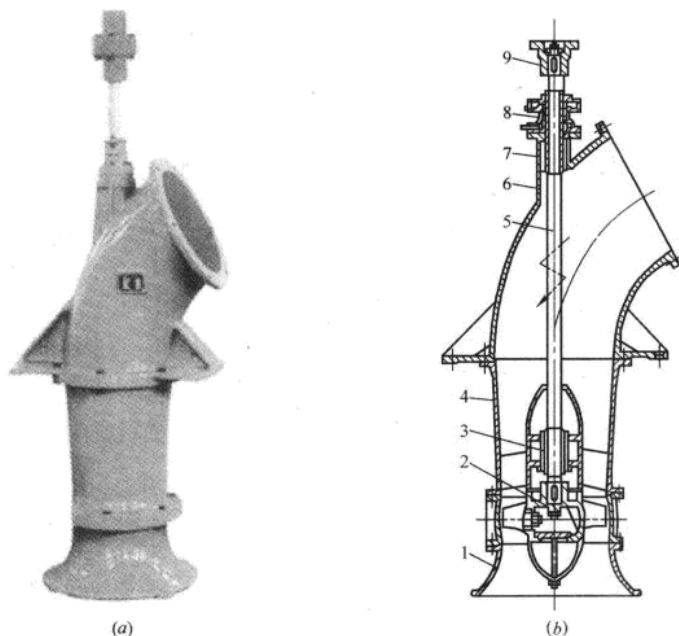
图 2-13 立式轴流泵
