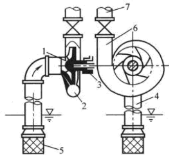
图 2-1 单级单吸式离心泵的构造
