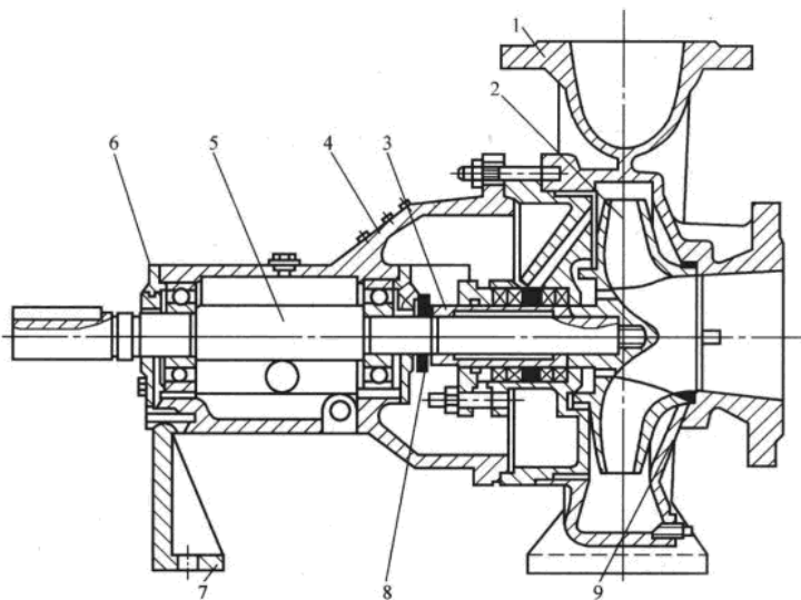
图 2-2 单级单吸式离心泵
