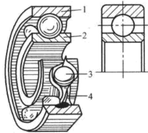
图 2-9 向心球轴承
