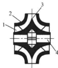
图 2-4 双吸式叶轮
