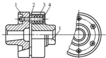
图 2-10 圆柱销弹性联轴器
