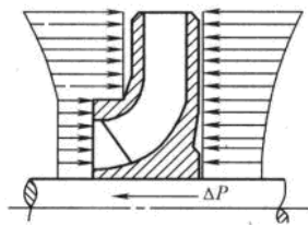
图 2-12 轴向推力
