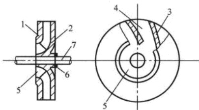
图 2-3 单吸式叶轮
