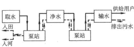
图 1-2 给水排水系统基本工艺流程
