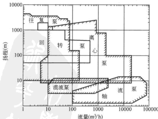
图 1-3 常用泵的使用范围
