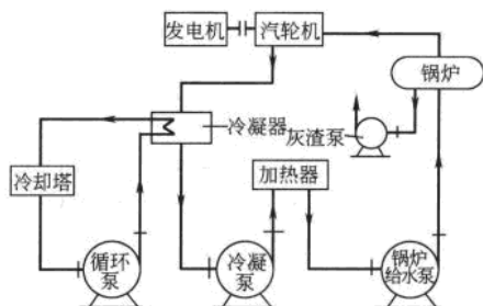
图 1-1 泵在火力发电厂中的应用示意图
