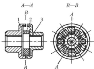
图 2-11 爪形弹性联轴器
