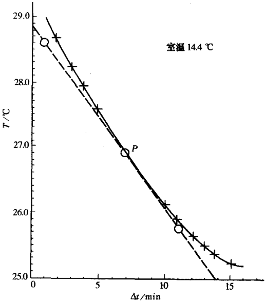
图 2 铝圆柱体散热曲线
