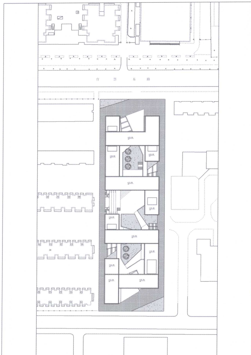
总平面图 1:2000
