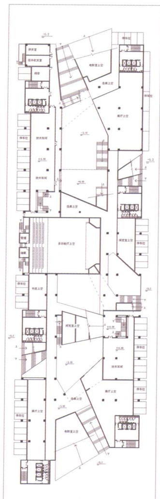
标高+1.00处平面图 1:200
