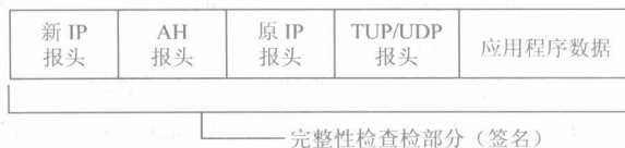
图1 ESP 报头形式
