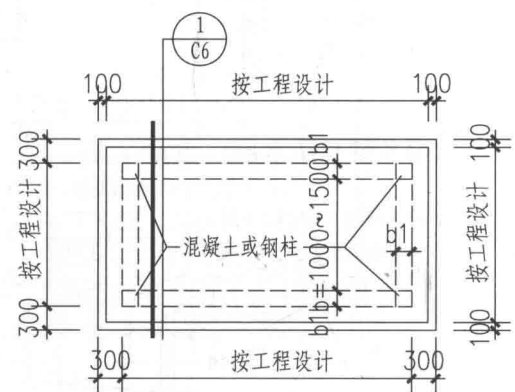
⑧ 种植土混凝土板平面图
