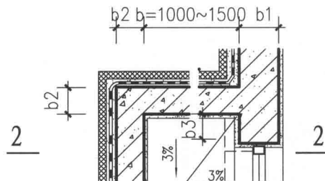
2 窗井平面示意图 (有防水层)
