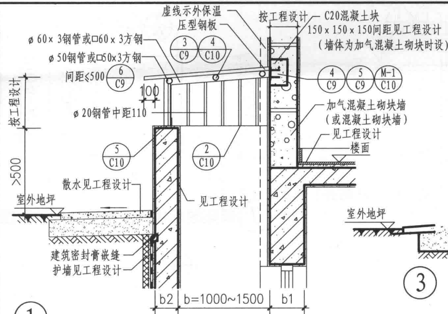
1 (窗井壁有防水层)
