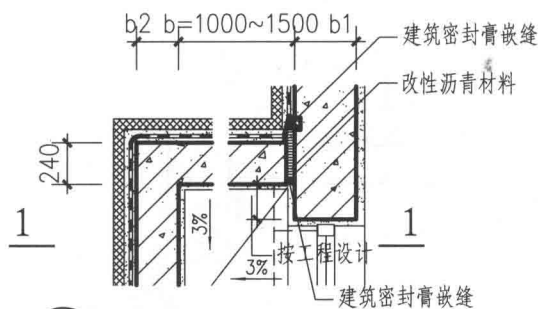
1 窗井平面示意图 (有防水层)
