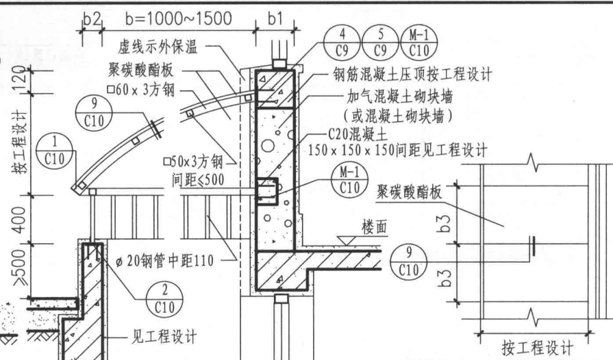
聚碳酸酯板窗井顶部局部平面
