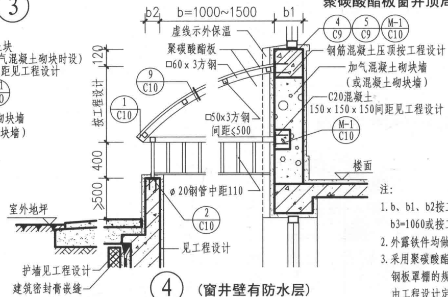
聚碳酸酯板、压型钢板窗井顶部详图
