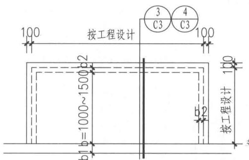
② 聚碳酸酯板平面图
