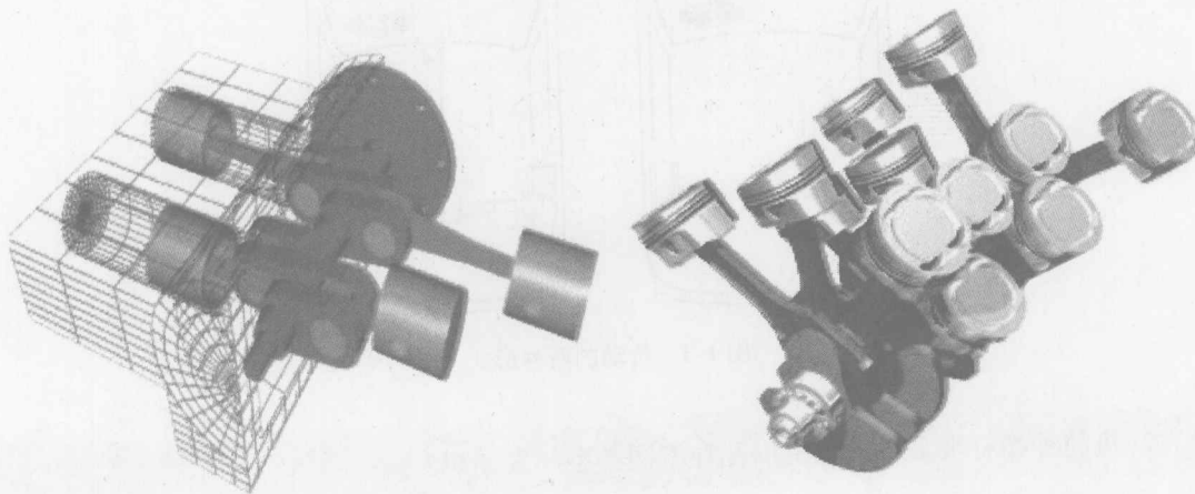
图 1-6 发动机的排列方式 (2)
