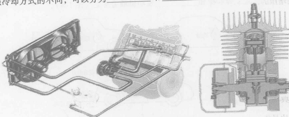
图 1-7 发动机的冷却方式
