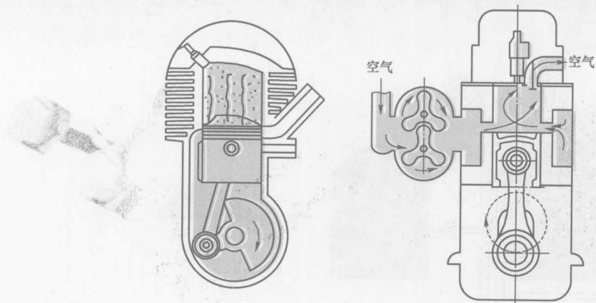
图1-9 发动机的进气
