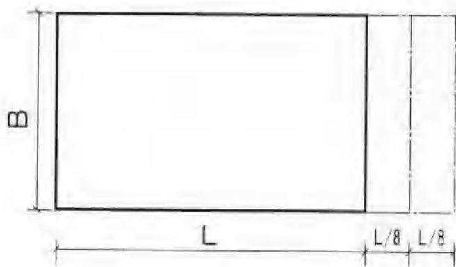
图 1-12 图纸加长方法
