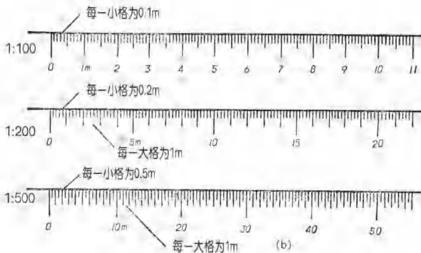
图1-6 比例尺及其识读
