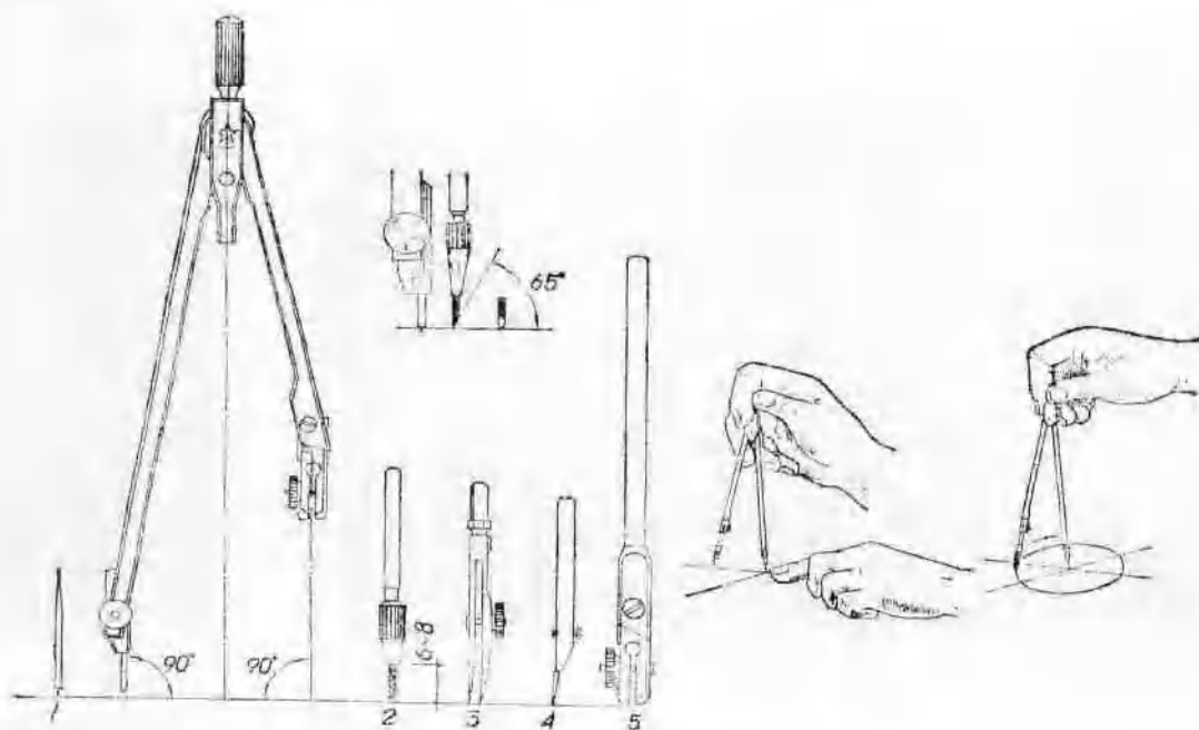
1. 钢针 2. 铅笔插腿 3. 直线笔插腿 4. 钢针插腿 5. 延伸杆
