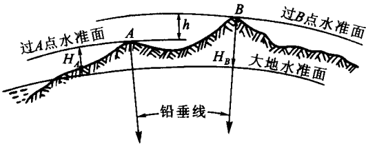
图 1-6 点的高程
