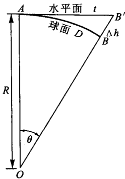
图 1-7 地球曲率的影响
