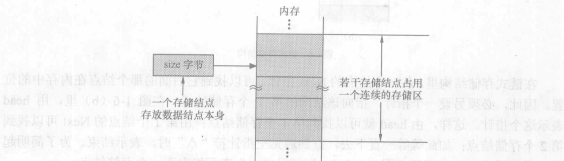
图 1-5 顺序存储结构
