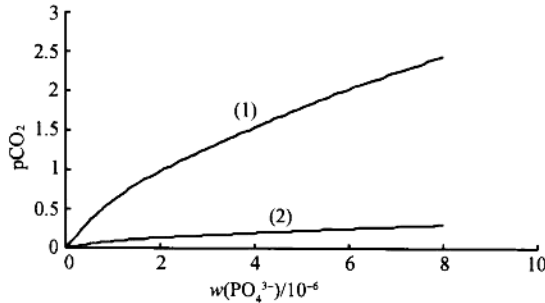
图 3 海水中 \text{pCO}_2 与 \text{PO}_4^{3-} 之间的消长关系
