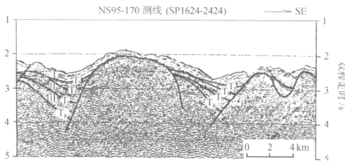
图 2 南沙海域地震剖面选段 (据姚永坚等, 1998)
