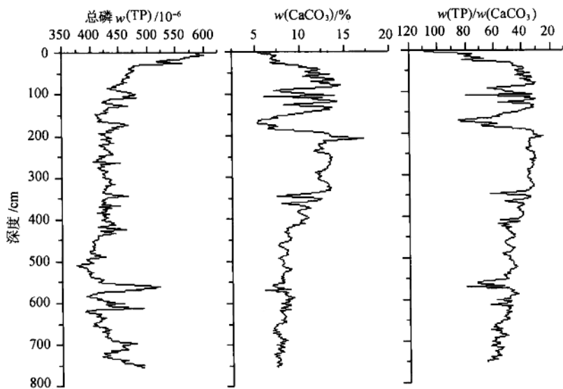
图1 南海北部陆坡沉积物中总磷与碳酸钙含量随深度变化的负相关性
