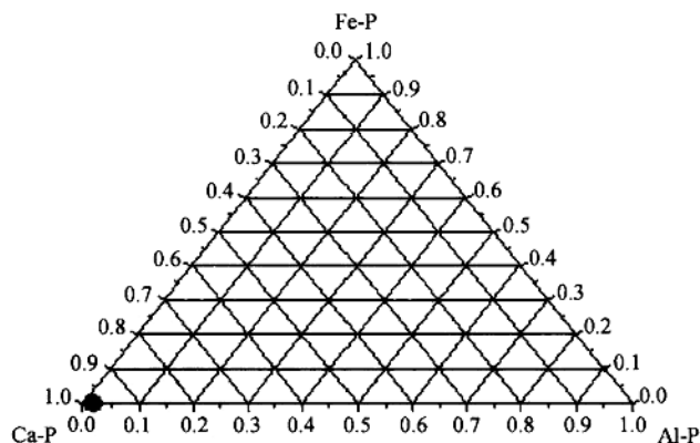
图2 沉积物中不同结合态磷(Ca-P, Fe-P, Al-P)的三角相图
