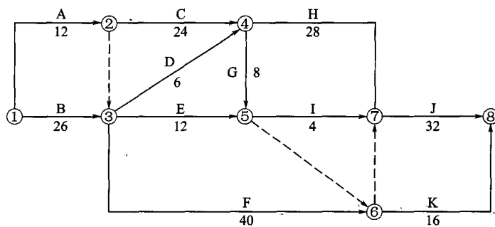
图 1-1 工程网络图
