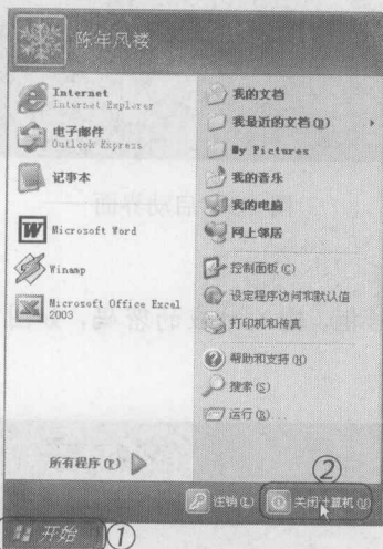
图 1-6 单击按钮
