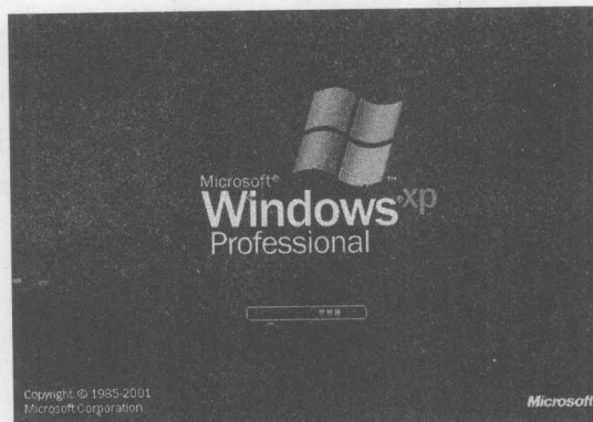
图 1-3 启动界面
