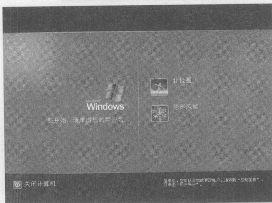
图 1-4 选择用户
