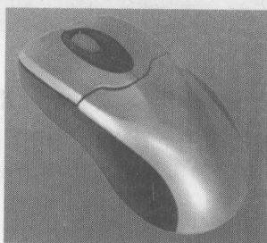
图 1-16 3D 鼠标
