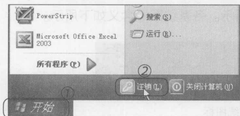
图 1-8 选择命令
