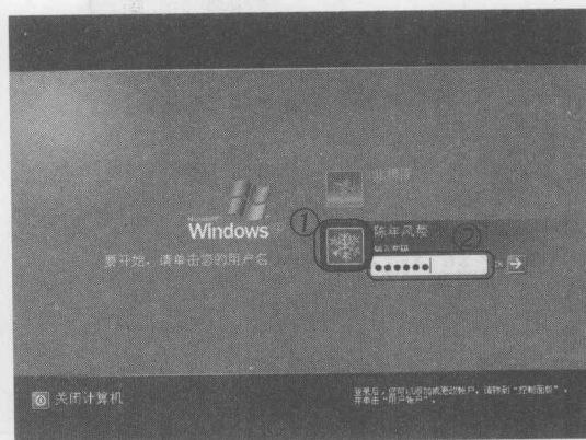
图 1-5 输入密码
