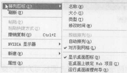
图 1-13 排列图标
