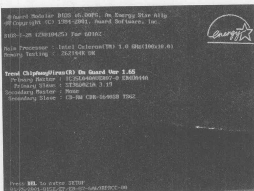
图 1-2 开始自检
