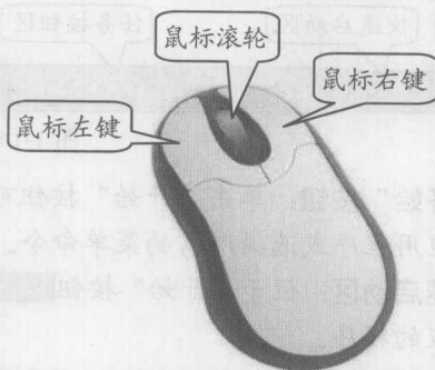
图 1-17 光电鼠标
