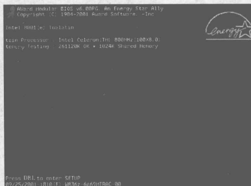
图 1-1 计算机自检
