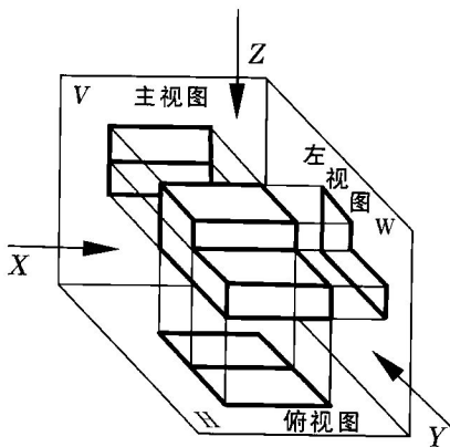
图2-6 三视图的形成
