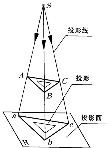
图2-1 中心投影法
