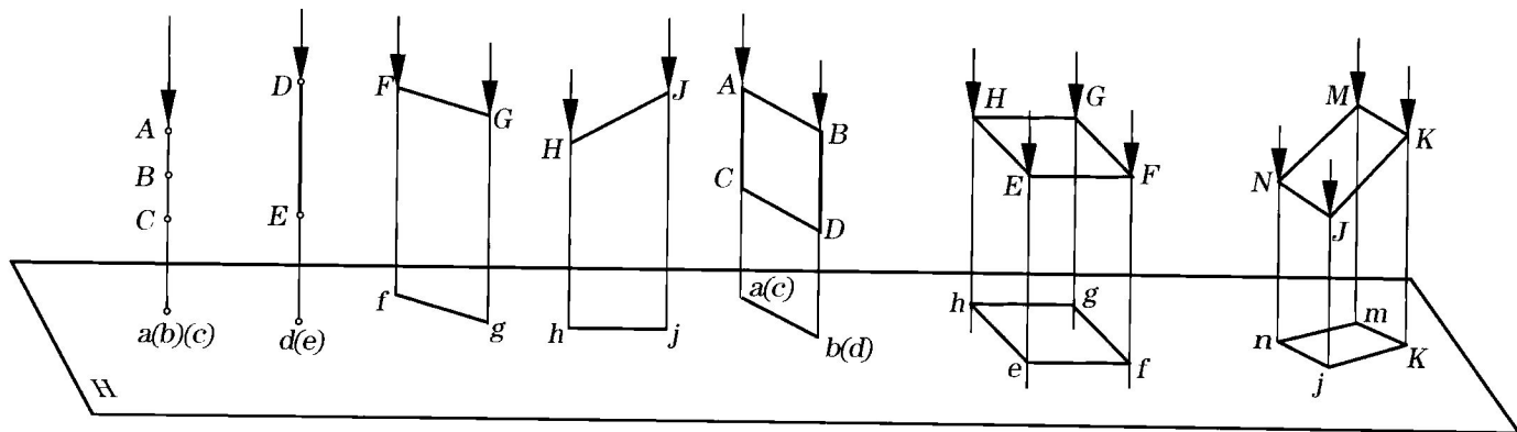
图2-3 点、直线和平面的正投影特性
