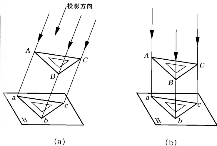
图2-2 平行投影法
