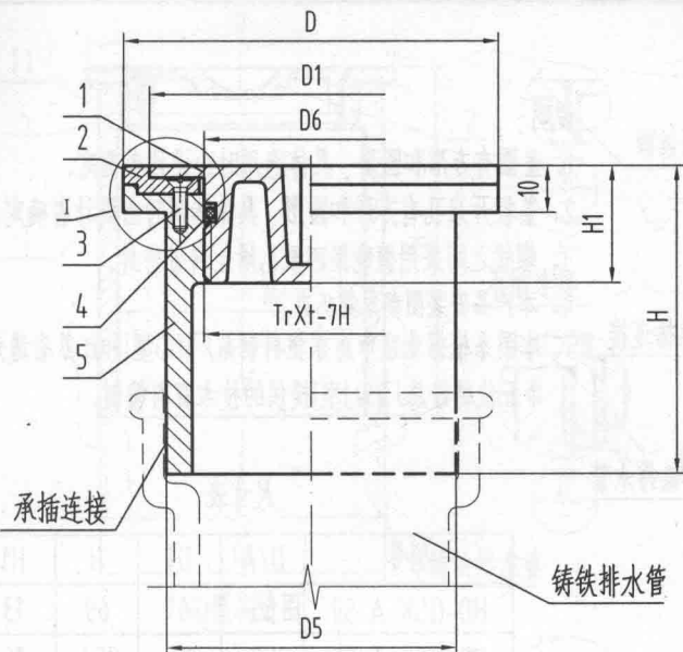
构造图
