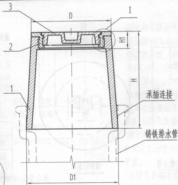
WJ型构造图
