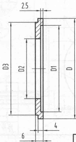
盖圈侧面图
