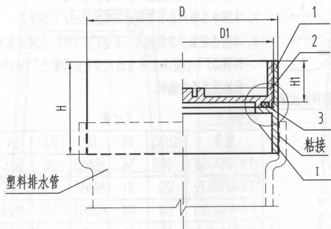
构造图
