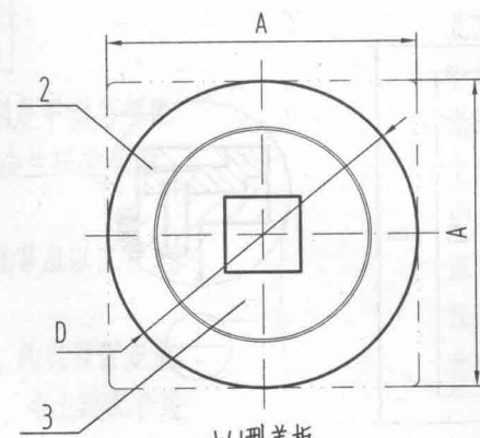
WJ型盖板
