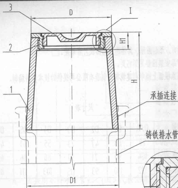
HD型构造图
