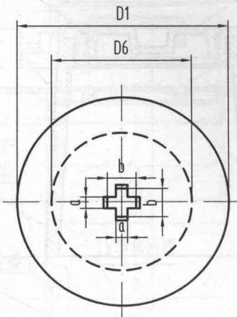
清扫口盖板
