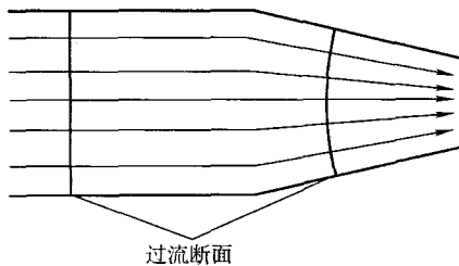
图 1-8 过流断面
