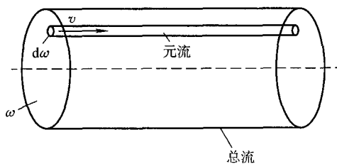
图 1-7 元流与总流
