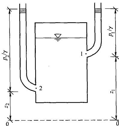
图 1-6 测压管水头
