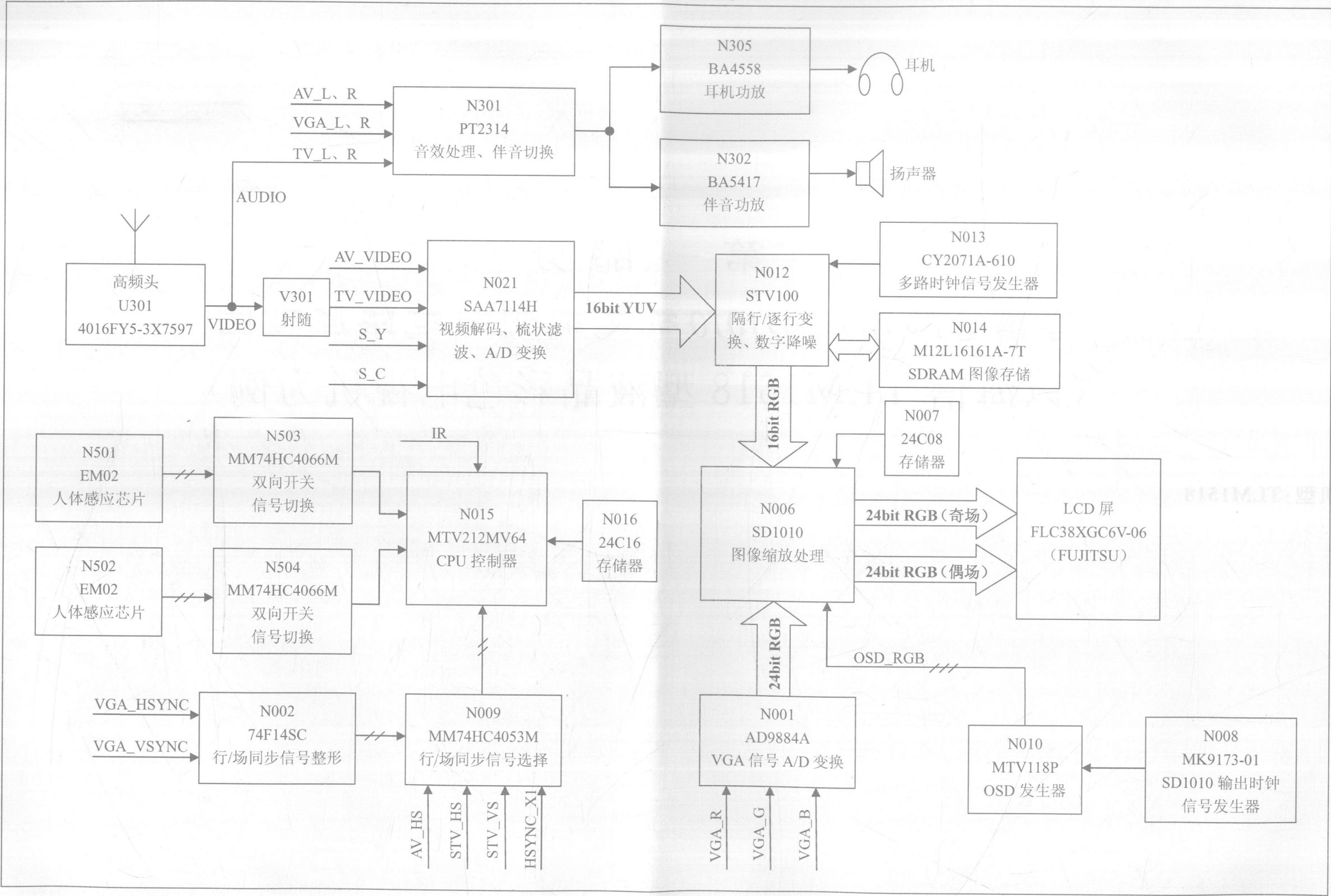
海信 TLM1518 型液晶彩色电视机电路原理图(1/9)——整机电路框图
