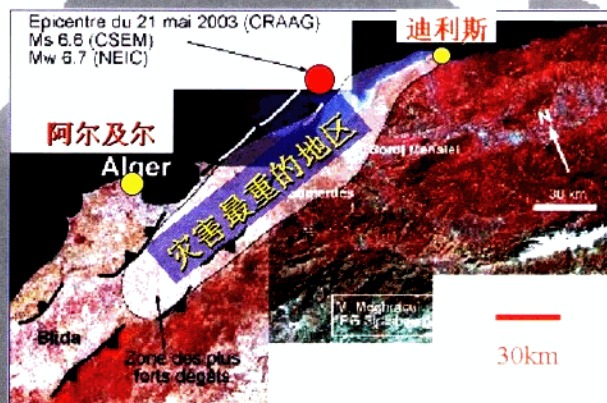
5月21日阿尔及利亚6.9级地震震中位置图
