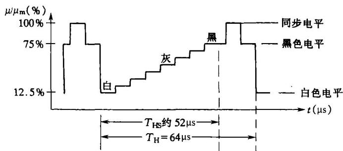
图 1.9 八级灰度图像一行的视频电视信号波形
