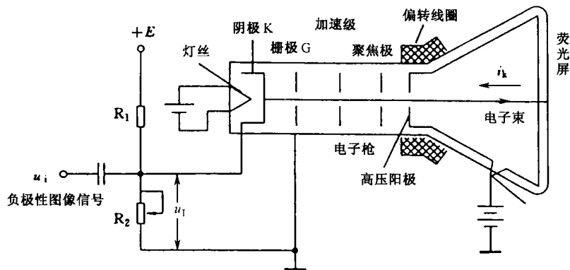
图 1.5 黑白显像管结构示意图
