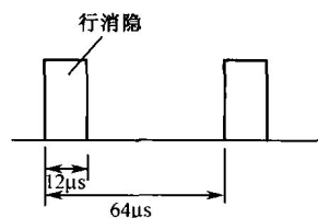
图 1.10 行消隐信号
