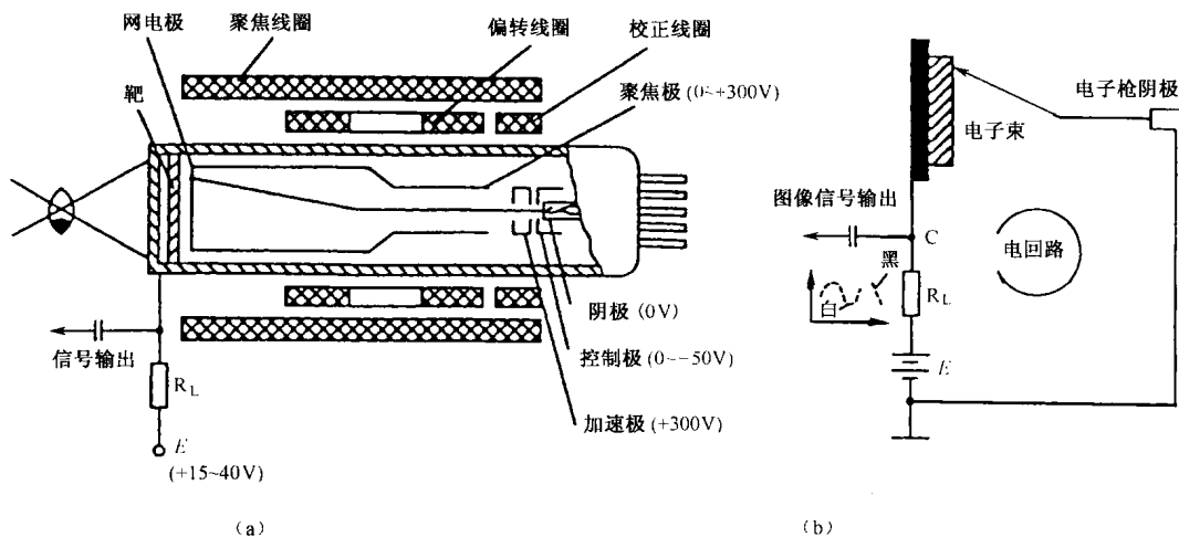
图 1.4 摄像管的光—电转换原理
