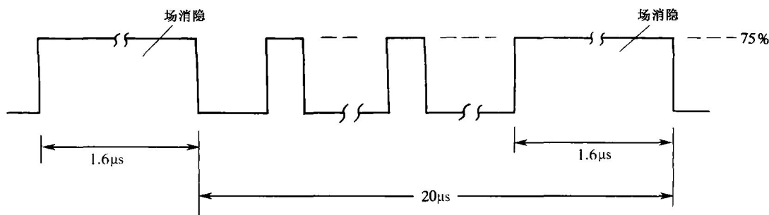
图 1.11 场消隐信号
