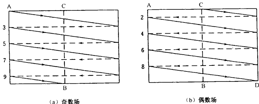
图 1.7 隔行扫描示意图
