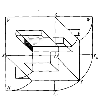
图 1-5 三个投影面的展开
