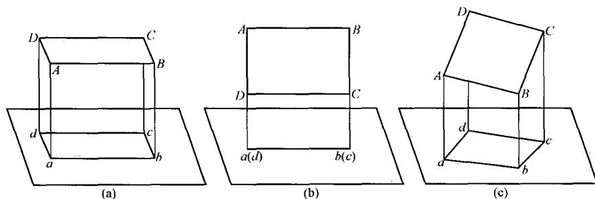
图 1-2 正投影规律
