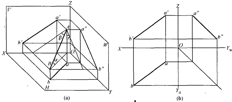
图 1-7 一般位置直线的投影 (a) 直观图; (b) 投影图
