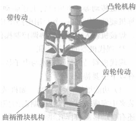
图 0-3 机构
