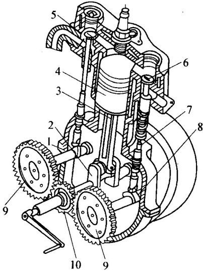
图 0-2 单缸四冲程内燃机
