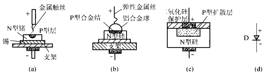
图 1-2-2 二极管的结构与符号
