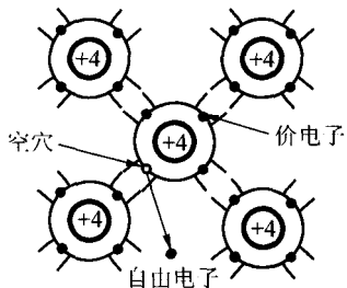
图 1-1-3 本征激发示意图
