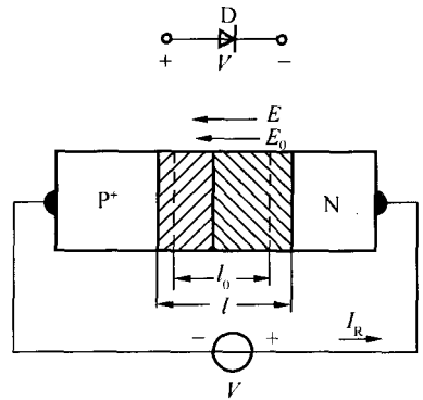
图 1-2-4 PN 结反向偏置
