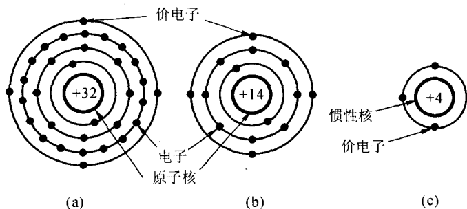
图 1-1-1 锗和硅原子结构模型
