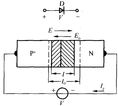
图 1-2-3 PN 结正向偏置
