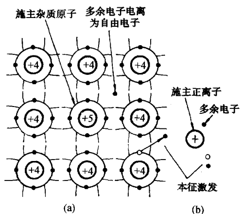
图 1-1-4 N 型半导体结构示意图
