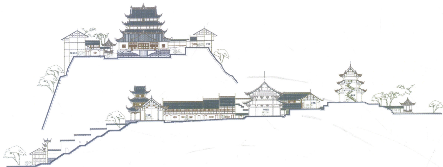
宝轮寺保护修复规划与设计场地剖面图
