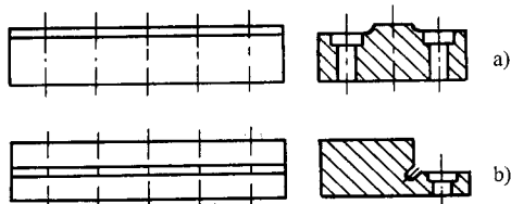
图 6.1-1 减小螺钉压紧变形对导轨精度的影响
