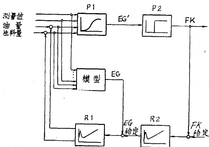
图4 WDK调节系统方案。
