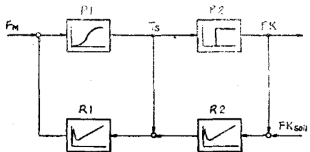
图3 WDK调节系统的设想方案
