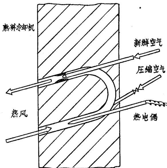
图1 二次空气温度测点的剖面图
