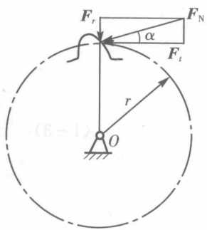
图 1-15 力矩的计算
