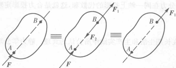
图 1-6 加减平衡力系公理
