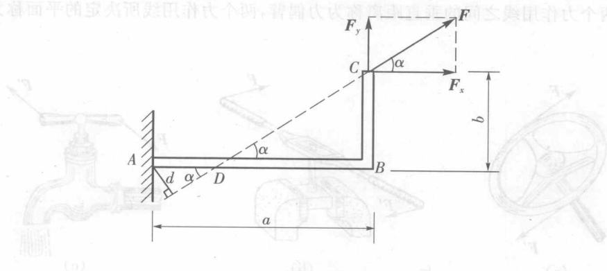
图 1-14
