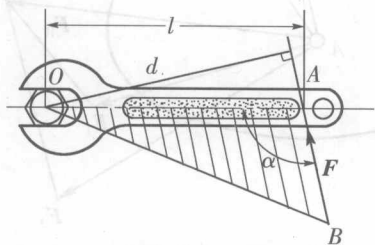
图 1-12 力对点之矩
