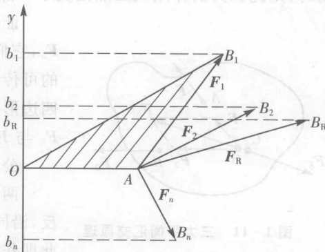
图 1-13 合力矩定理
