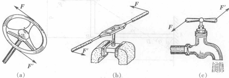
图 1-16 力偶的实例
