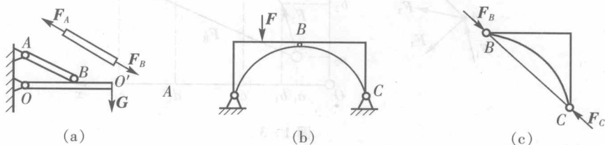
图 1-5 二力构件和二力杆
