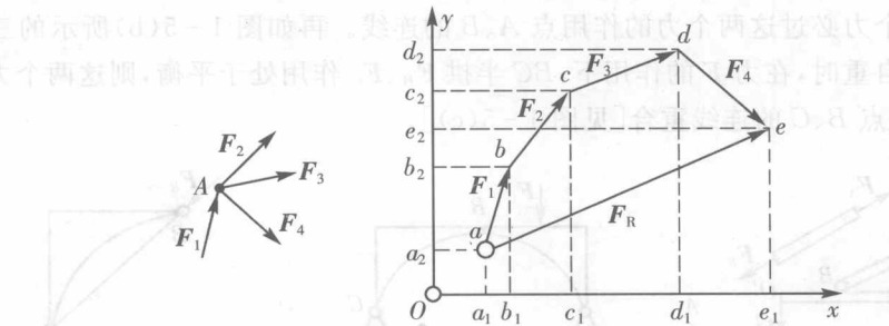
图 1-3
