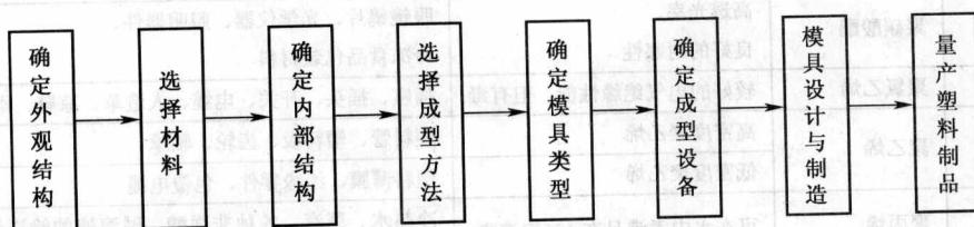
图 1-1 塑料制品的设计流程
