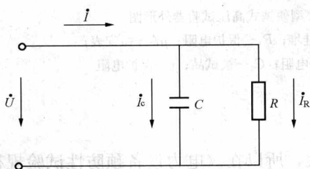
图 1-6 介质等值电路
