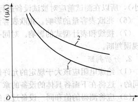
图 1-4 泄漏电流和时间的关系曲线
