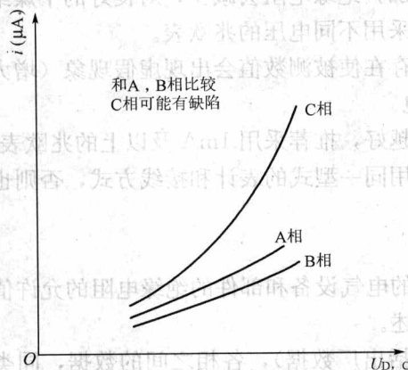
图 1-3 泄漏电流和电压的关系曲线
