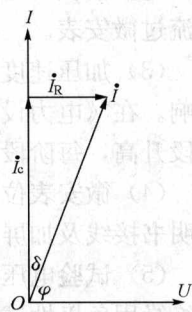
图 1-7 等值电路电流、电压相量图
