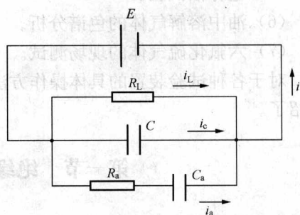
图 1-2 测绝缘电阻时的等值回路图
