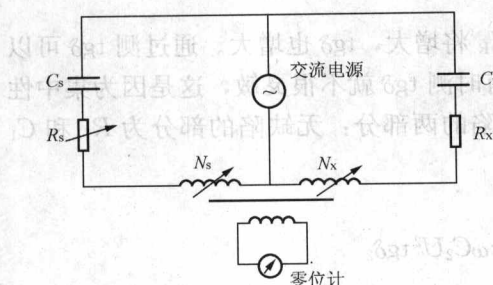
图 1-9 Biddle 功率因数 (PF)
