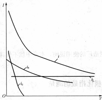
图 1-1 绝缘在直流电压下通过的电流
