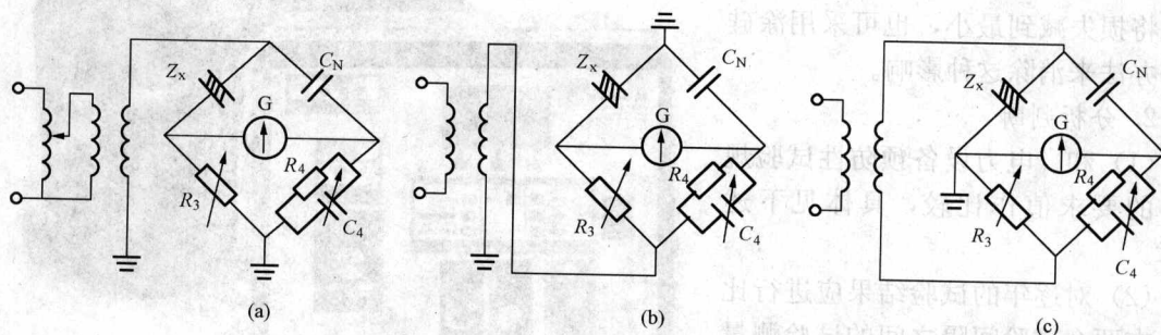
图 1-8 QS1 型西林电桥原理接线
