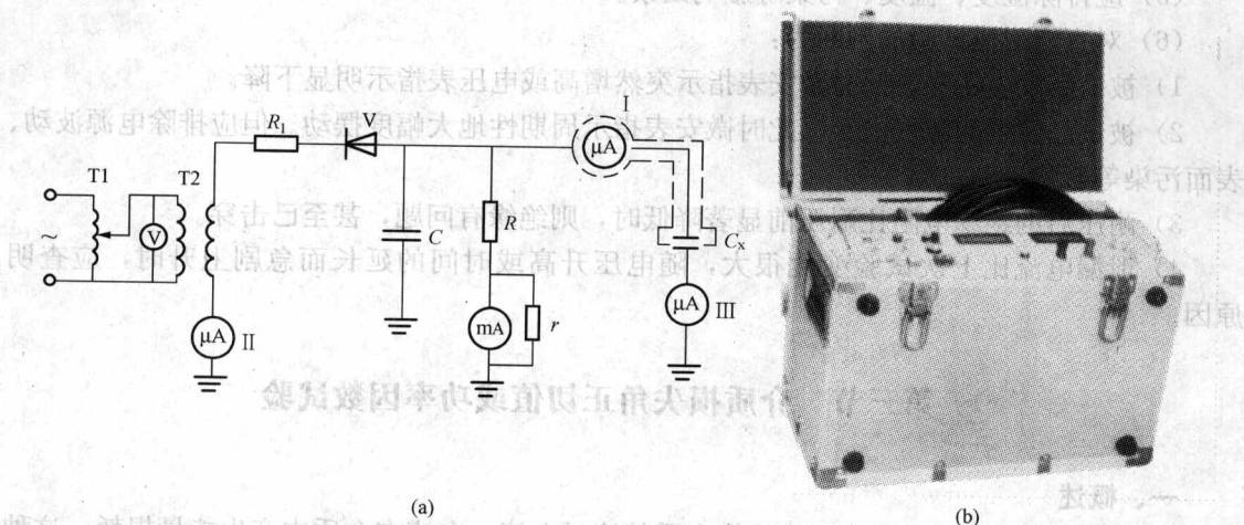
图 1-5 测量泄漏电流和直流耐压
