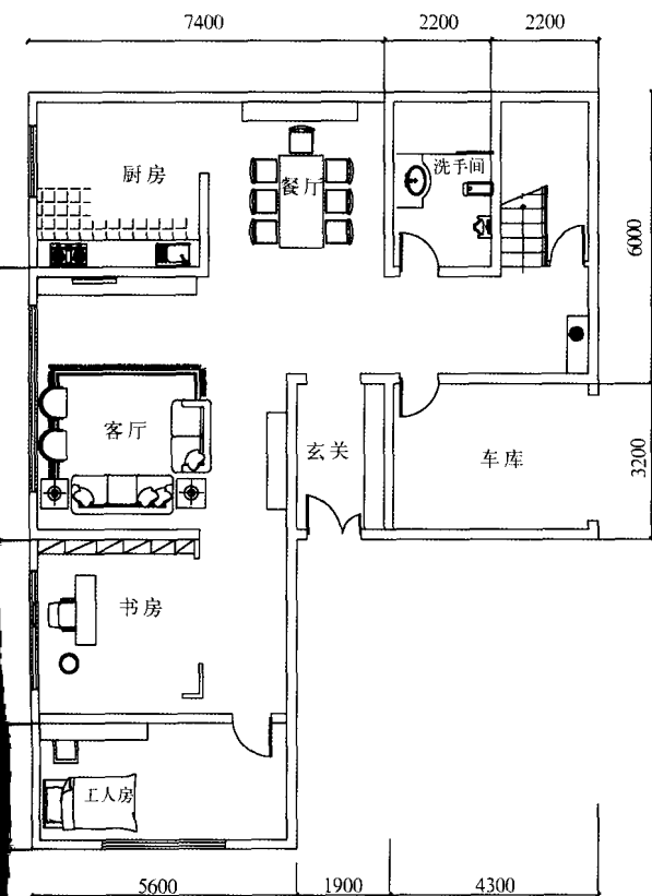
一层平面图
