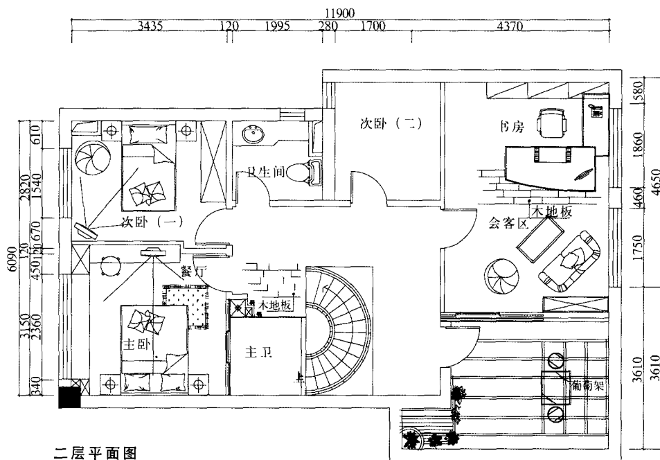
二层平面图
