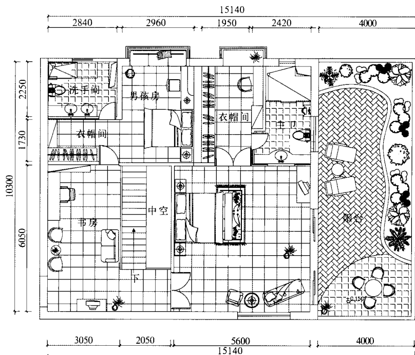
二层平面图
