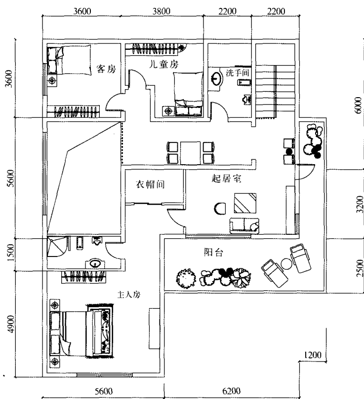
二层平面图
