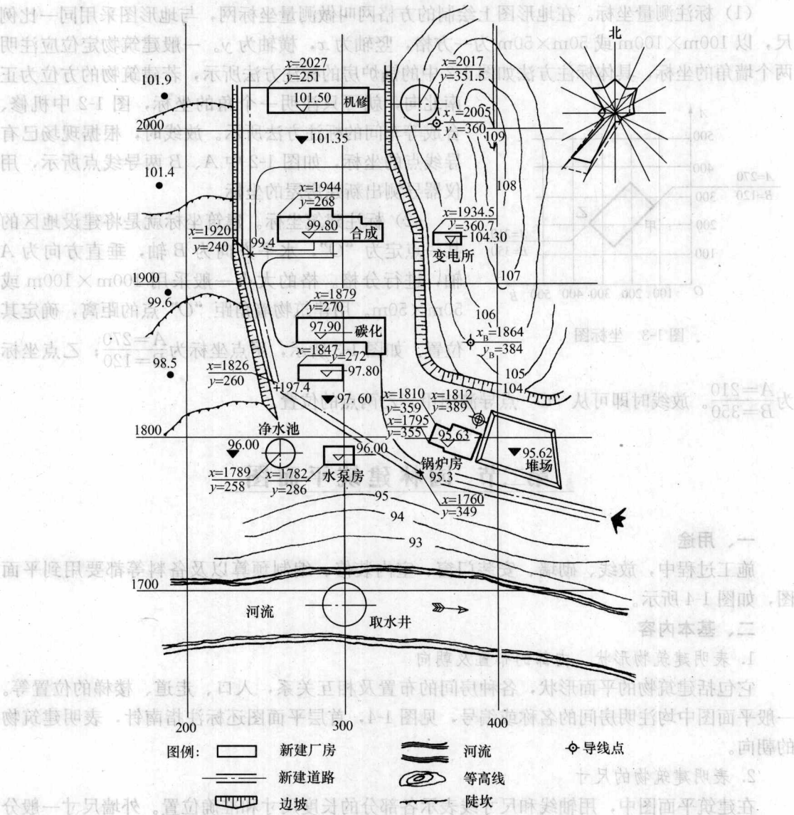
图 1-2 某厂总平面图
