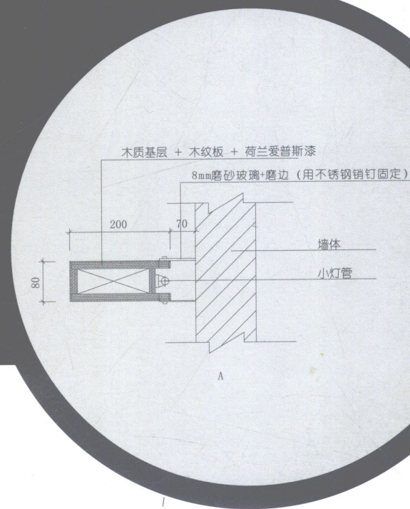
多功能木架与墙体连接图
