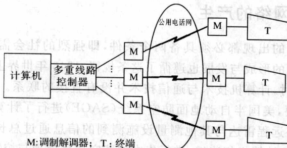
图 1-2 面向终端的计算机通信网
