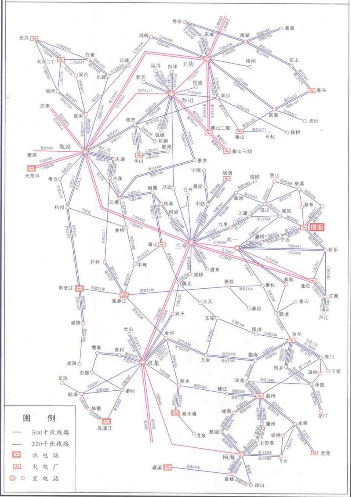
镇海发电厂与浙江电网 220~500 千伏电力系统接线示意图 (2005 年)
