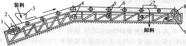
图 1-1 带式输送机
