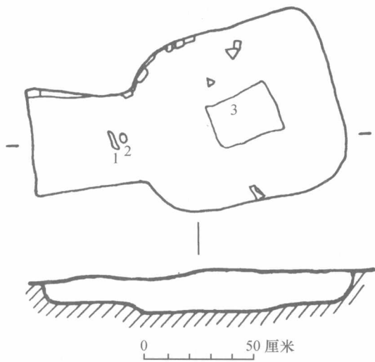
图五 Z2 平、剖面图
