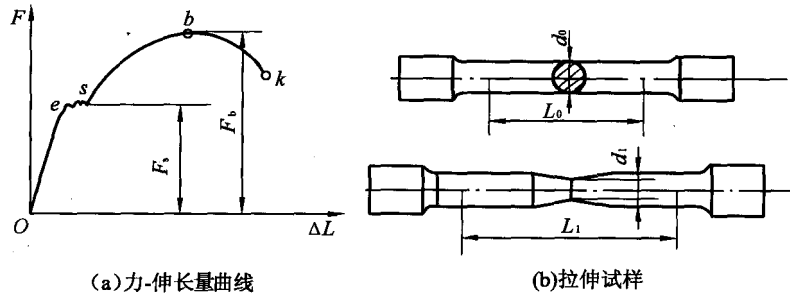
图 1-1 退火低碳钢的力-伸长量曲线和拉伸试样
