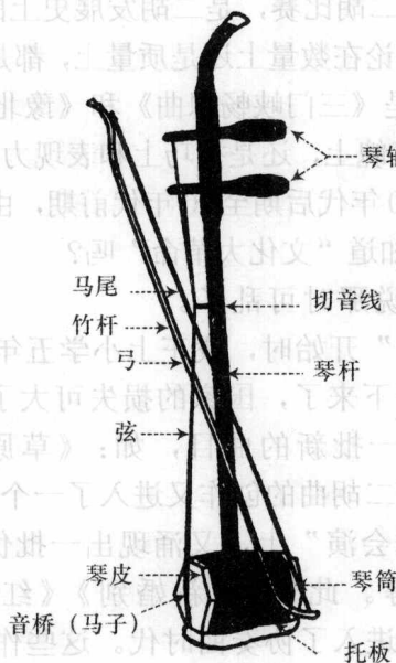
图1 二胡构造图
