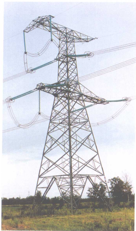
500千伏七台河—方正 —哈尔滨输电线路终端塔
