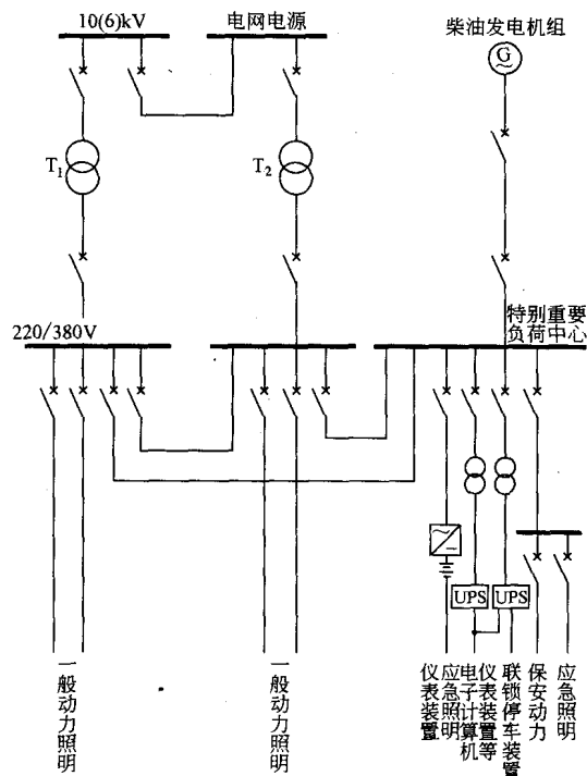
图 2.0.4 应急电源接线示例
