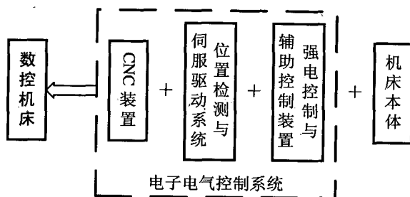
图 0.1.1 数控机床的组成框图(表示法 1)
