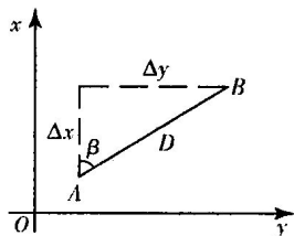
(1-1) 图 1-2 地面点的定位
