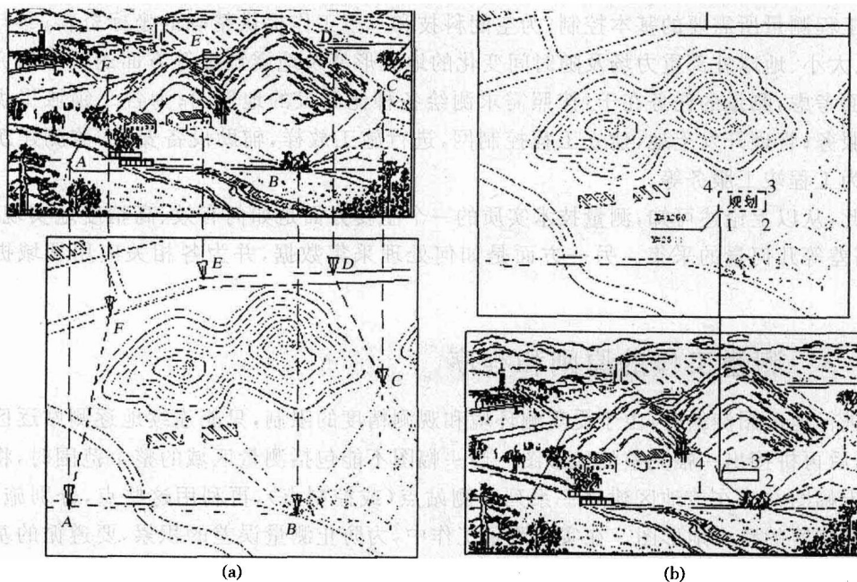
图 1-1 测定与测设的关系
