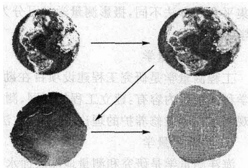
图 1-4 地球形状认识演变
