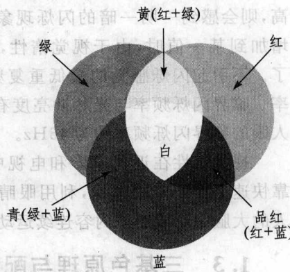
图 1.7 相加混色
