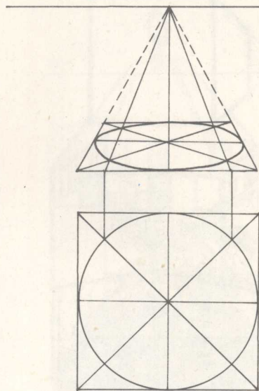
平置圆的透视
